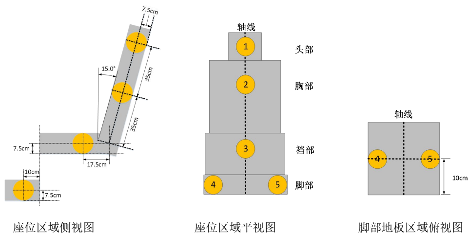
图 C.8 座位区域测试点位示意图
