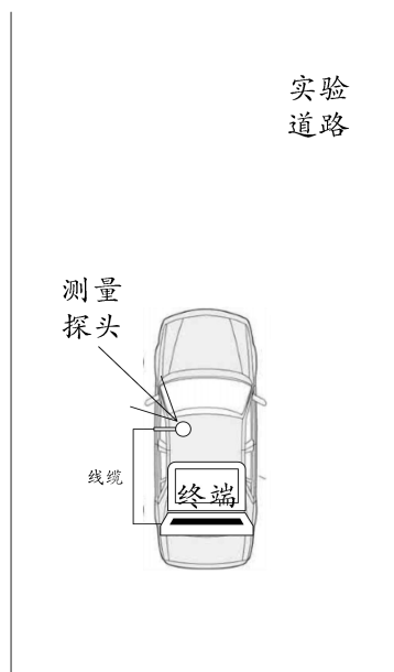
图 C.2 急加减速行驶工况测试布置图
