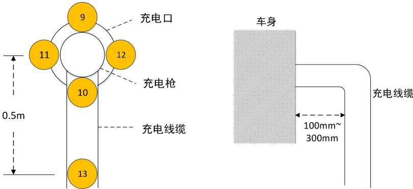
图 C.10 充电区域测试点位示意图
