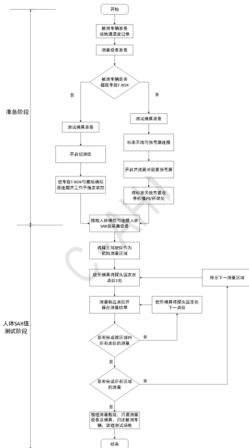
图 C.16 人体 SAR 值工况测试流程图
