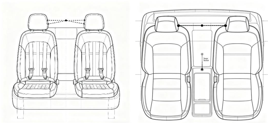
图 G.1 车内测温点位置示意图
