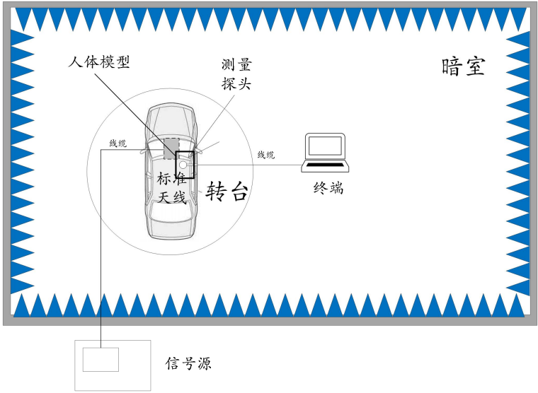
(b) 信号源+标准天线+人体模型
