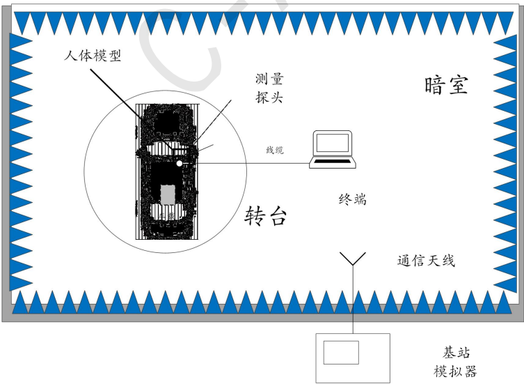
(a) 基站模拟器+车载 T-BOX+人体模型
