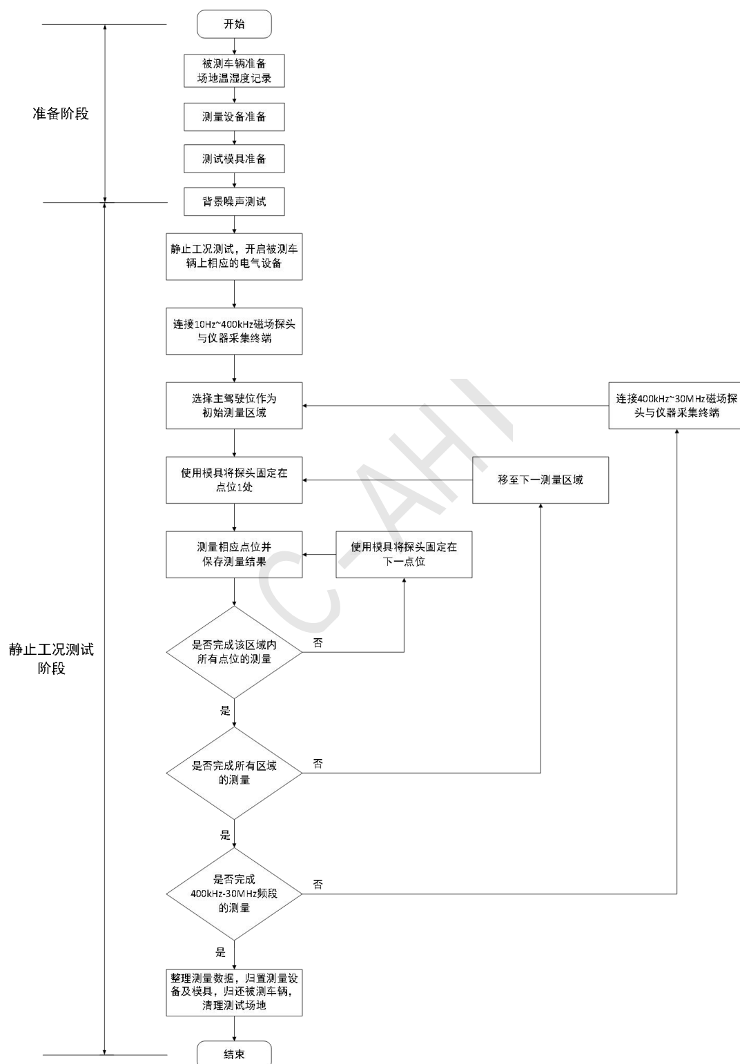
图 C.12 静止工况测试流程图
