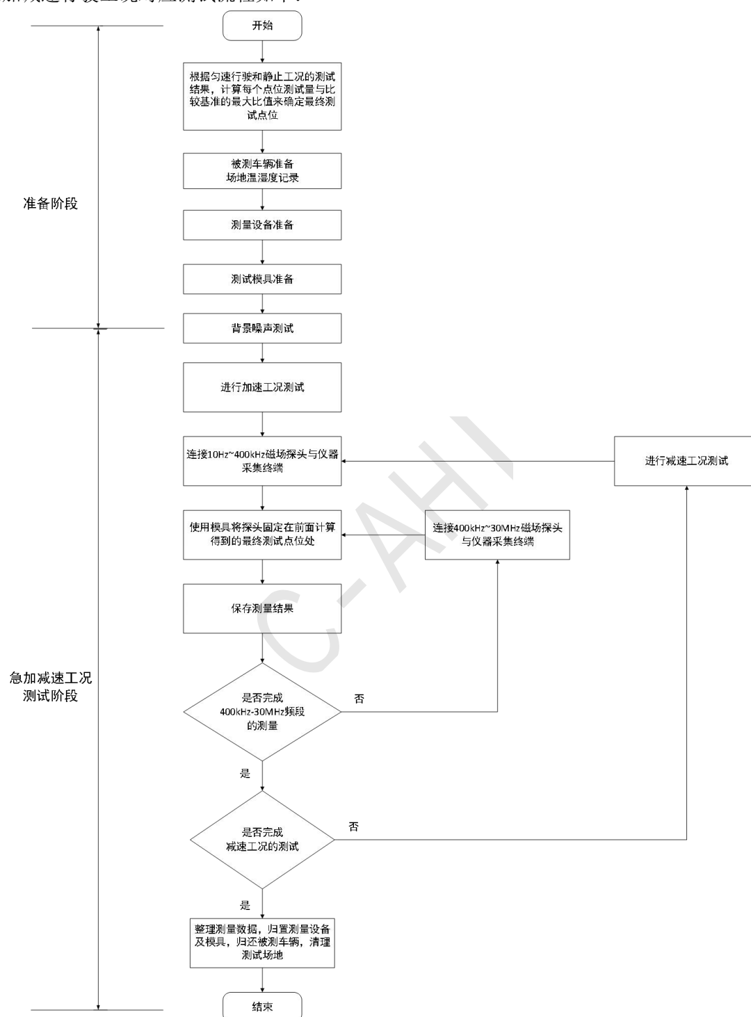
图 C.13 急加减速行驶工况测试流程图
