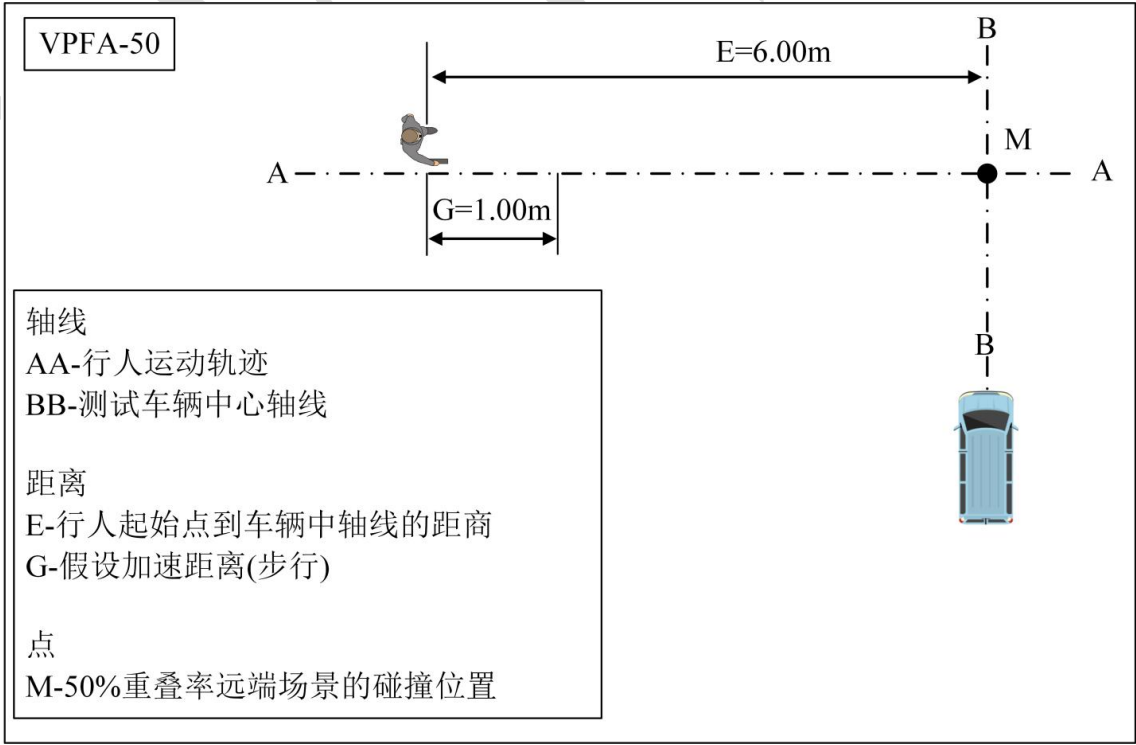
图 22 VPFA-50 工况
