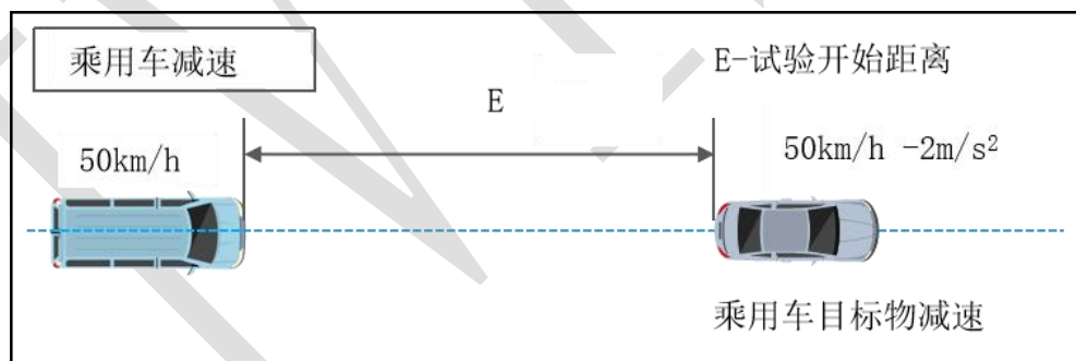
图 17 AEB 乘用车减速工况
