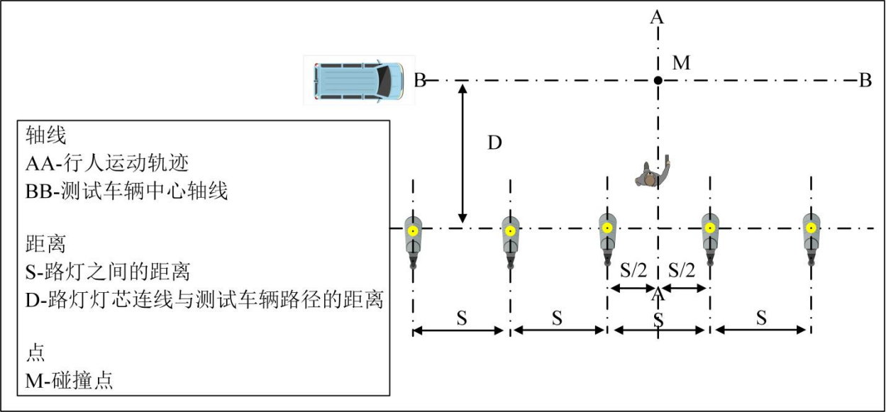
图 10 路灯安装位置
