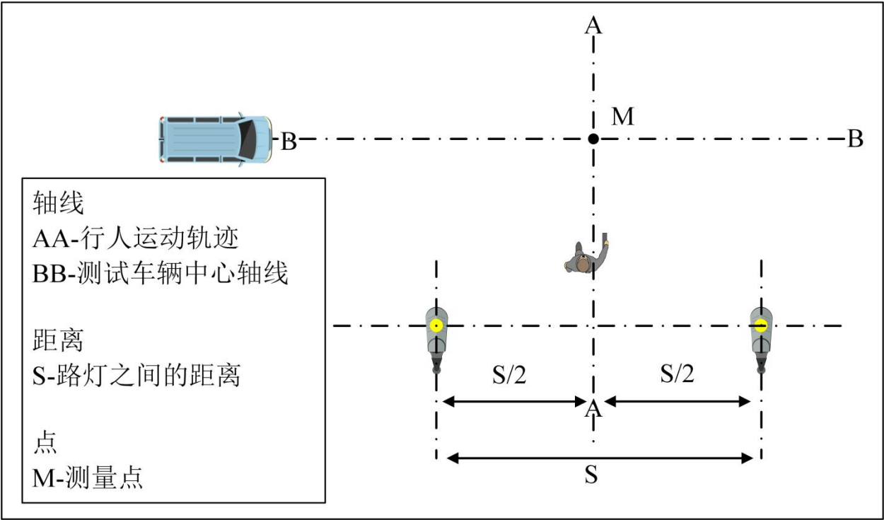
图 7 背景照度测量
