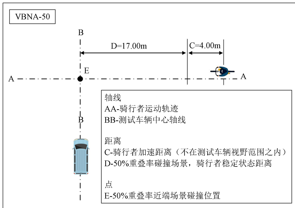
图 25 VBNA-50 工况
