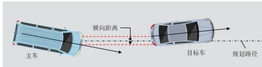
图 2 车对车横向距离
