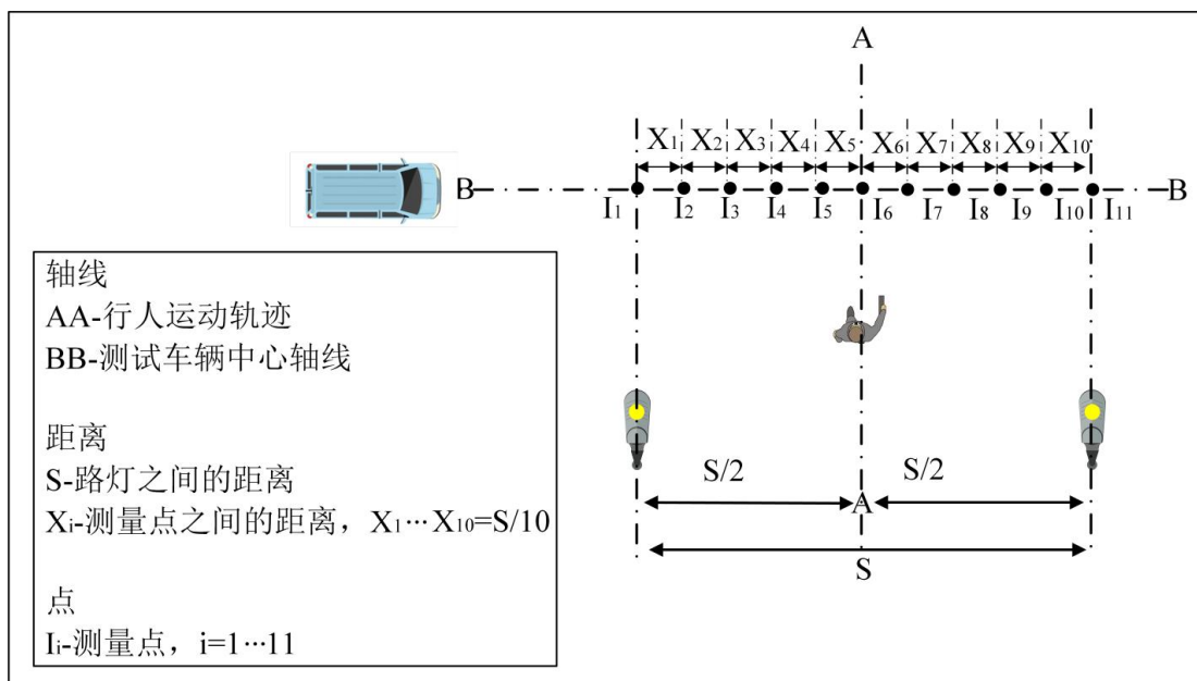
图 8 主车路径上的照度测量
