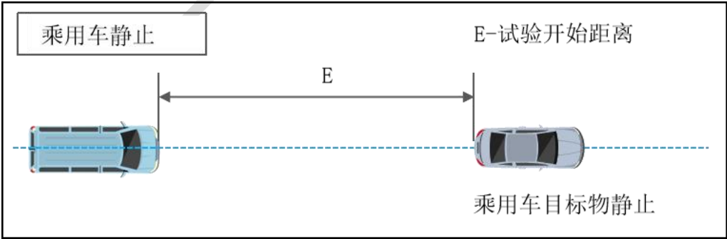
图 11 FCW 乘用车静止工况
