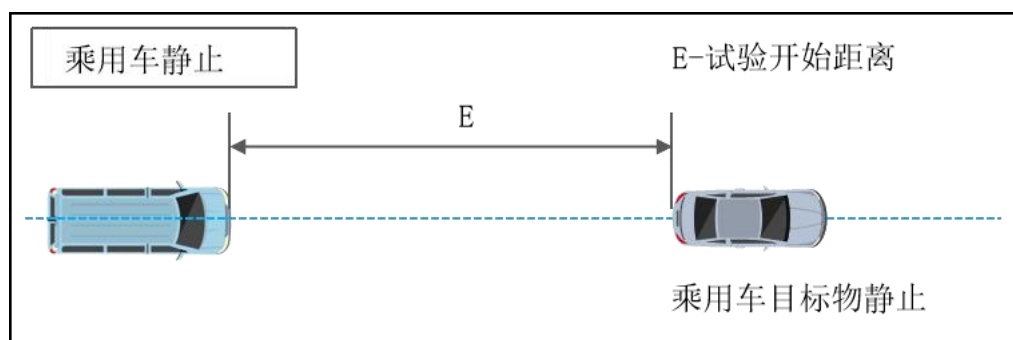
图 13 AEB 乘用车静止工况
