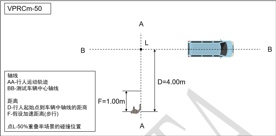
图 24 VPRCm-50 工况
