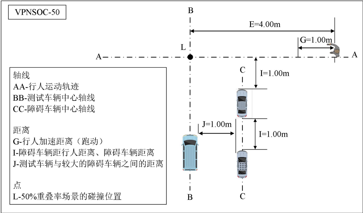
图 21 VPNSOC-50 工况
