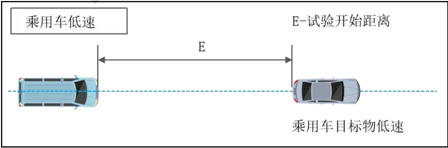
图 16 AEB 乘用车低速工况
