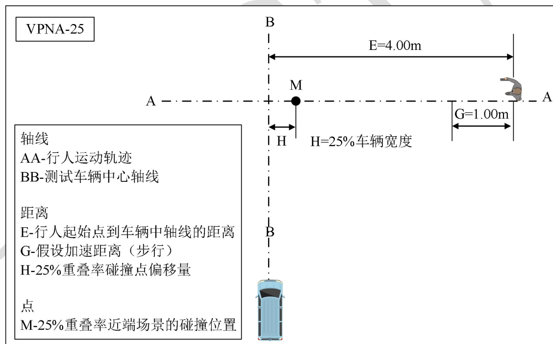
图 20 VPNA-25 工况
