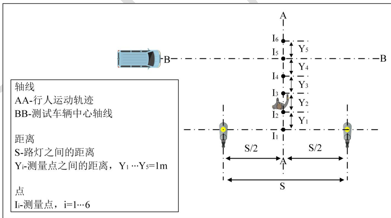
图 9 行人路径照度测量
