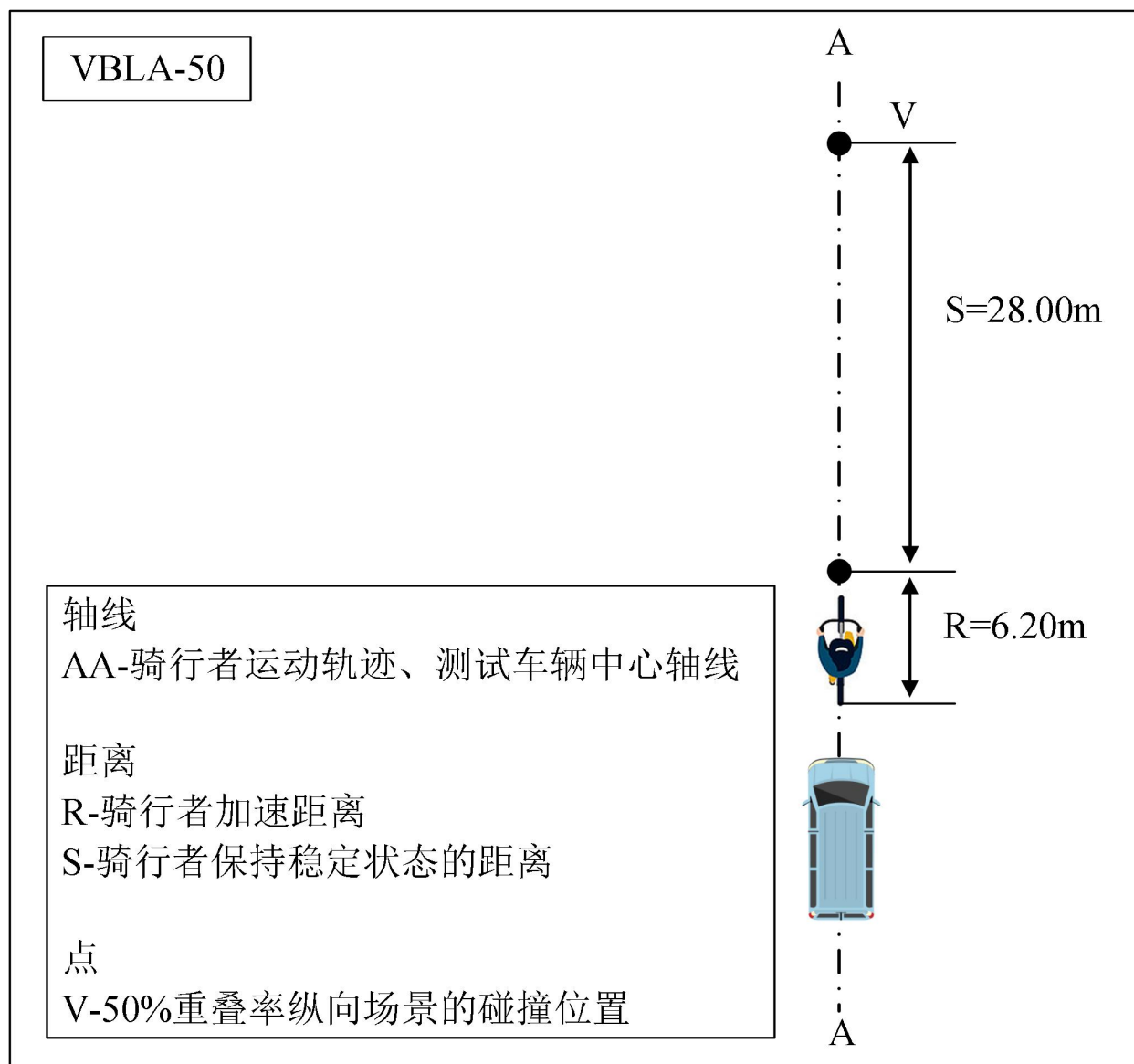
图 26 VBLA-50 工况
