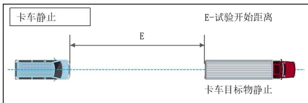
图 12 FCW 卡车静止工况
